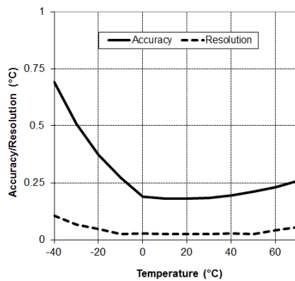
Graphik A: Interne Temperaturgenauigkeit und Auflösung
