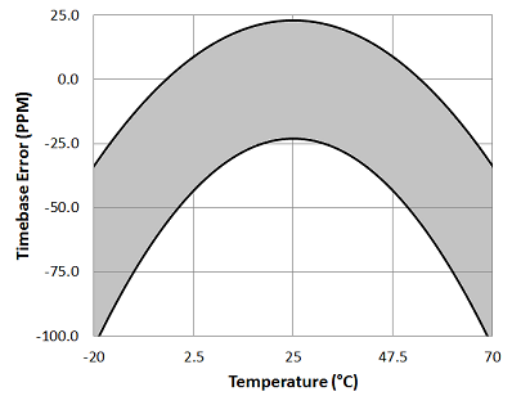
Graphik B: Zeitgenauigkeit
