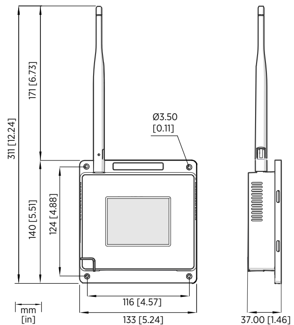
AP10 Abmessungen
