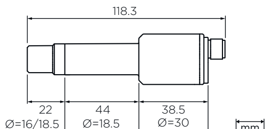
Abmessungen HPP271
