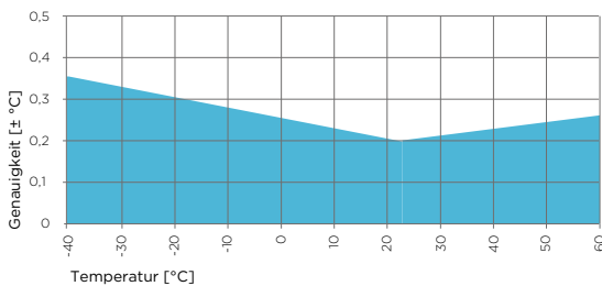
Genauigkeit der Temperaturmessung über den gesamten Messbereich
