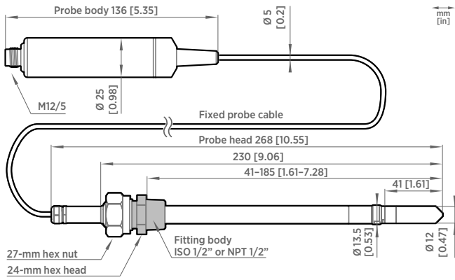
DMP8 dimensions
