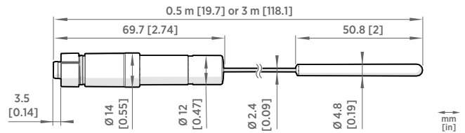
TMP115 dimensions
